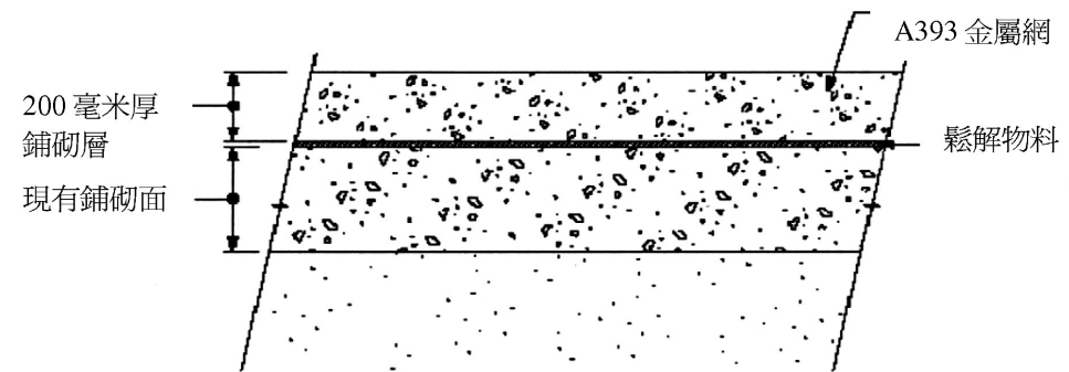
詳圖 1:20 B
